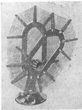
ANTENA DE CUADRO VARIABLE Con objeto de obtener propiedades direccionales, así como la de variar la inductancia del circuito de antena, se acaba de construir la que ilustramos en este grabado. Los dos enrollados, están instalados sobre dos marcos separados y pueden girar sobre la perilla especial que se encuentra allí. Estos enrollados están conectados en serie.
